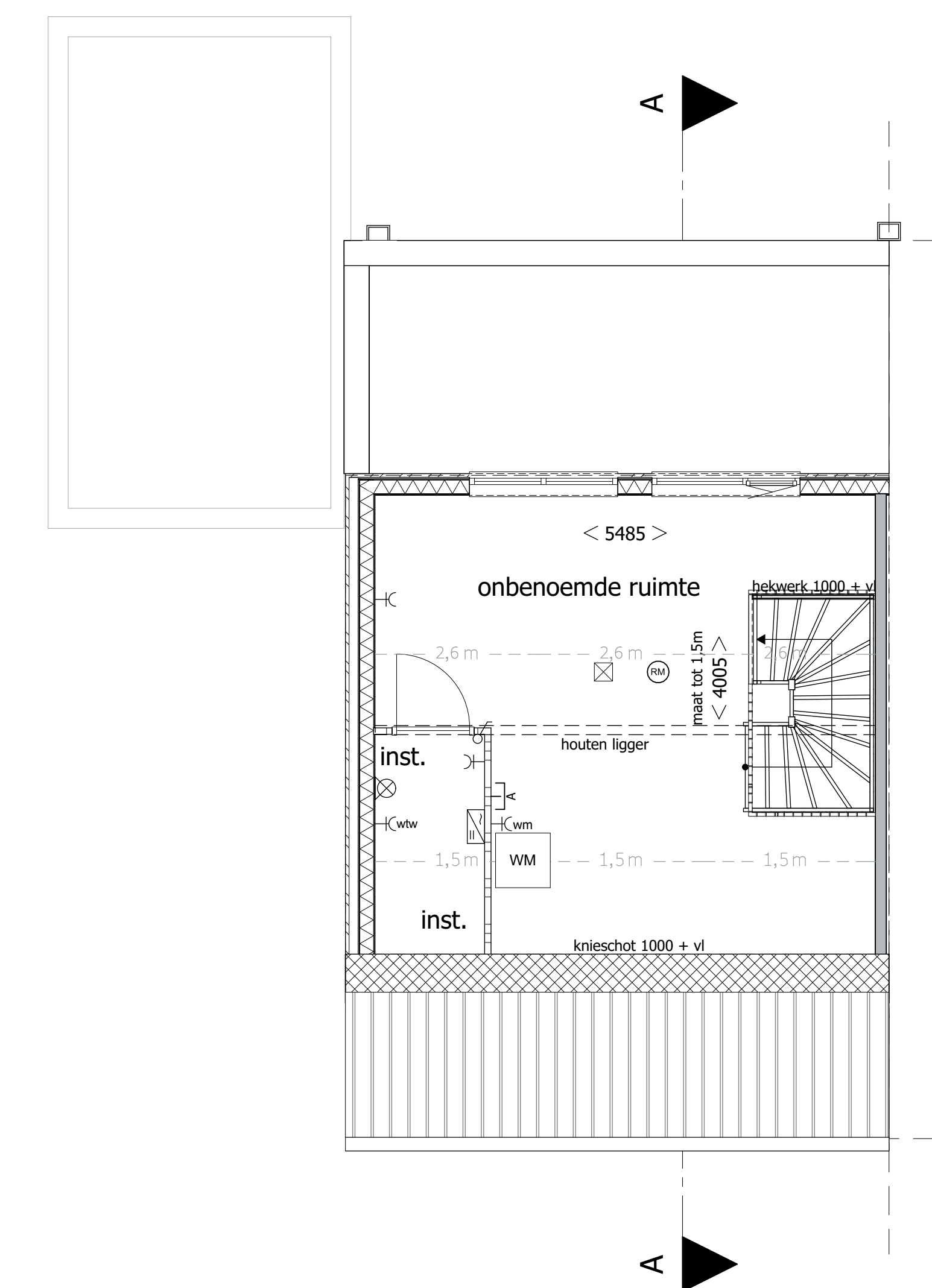
Verdieping 2 type G1
