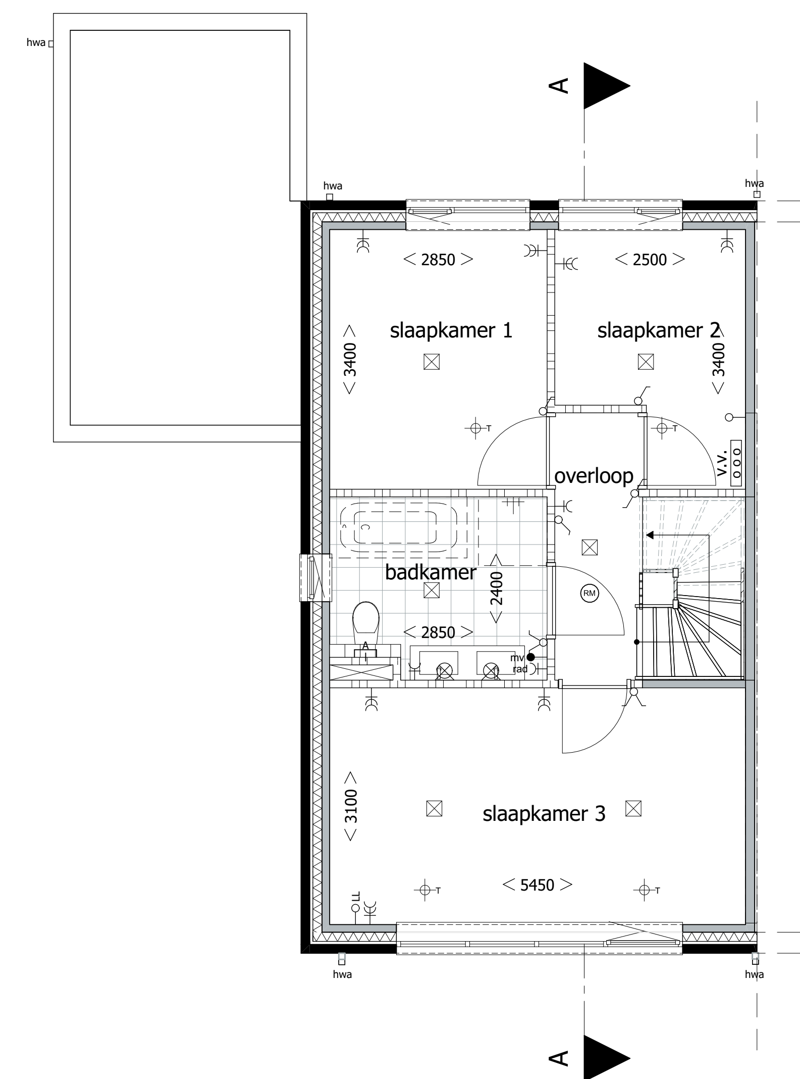
Verdieping 1 type G1
