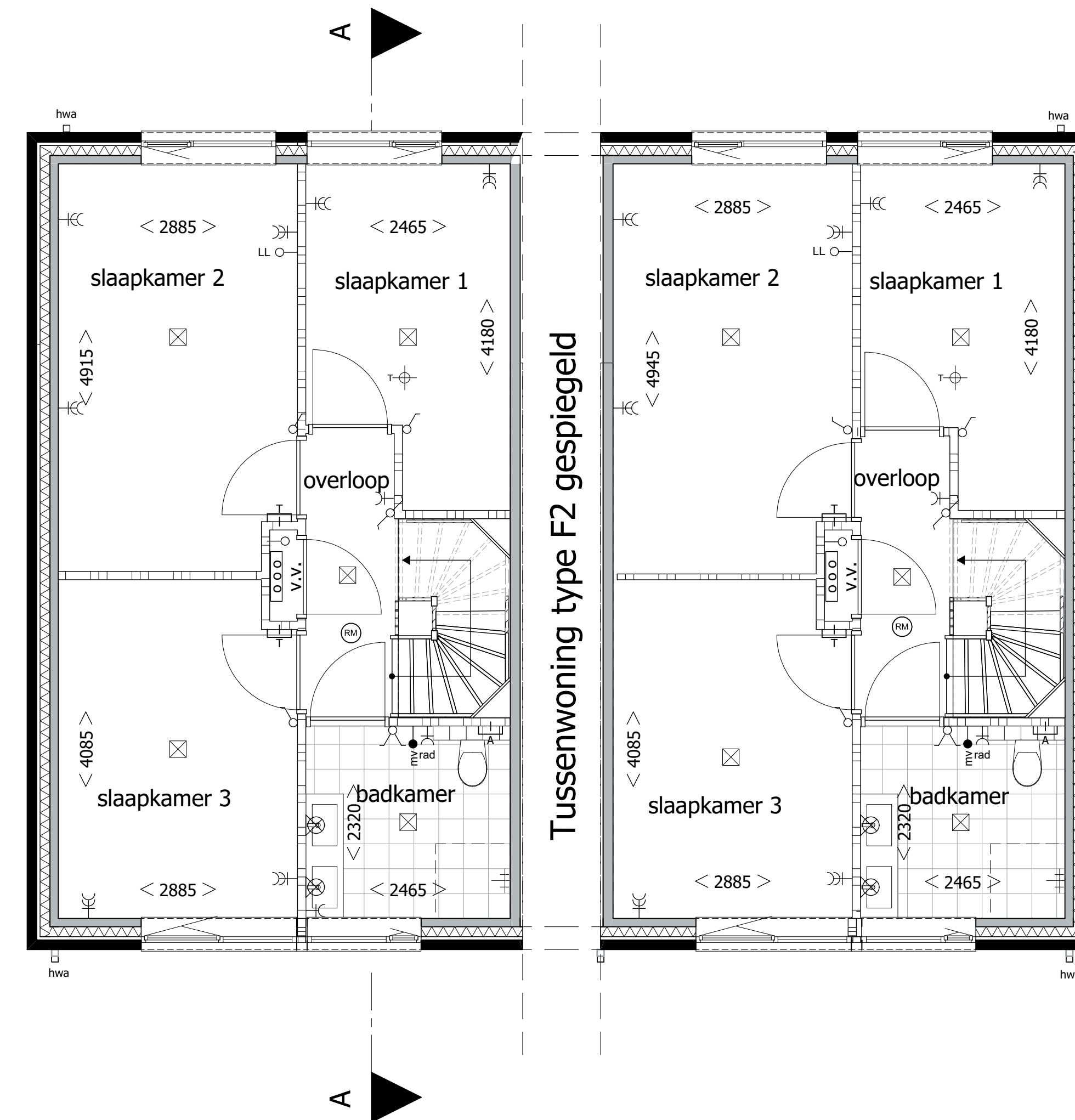
Verdieping 1 type E4 Verdieping 1 type E5 Bouwnummer 80 Bouwnummer 83
