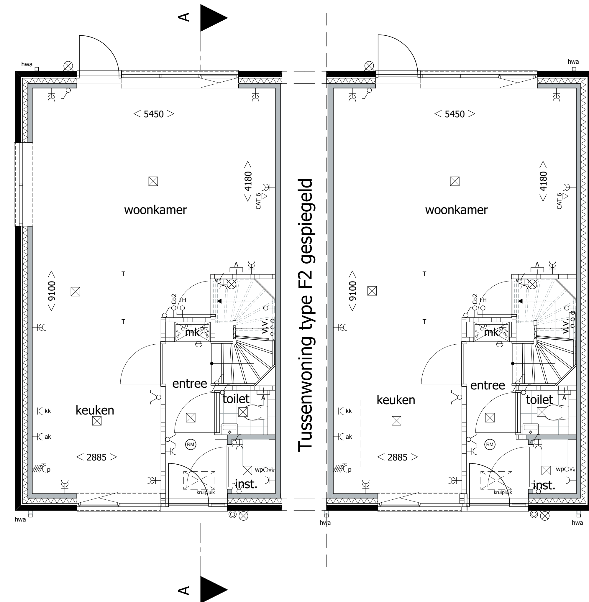
Begane grond type E4 Begane grond type E5 Bouwnummer 80 Bouwnummer 83
