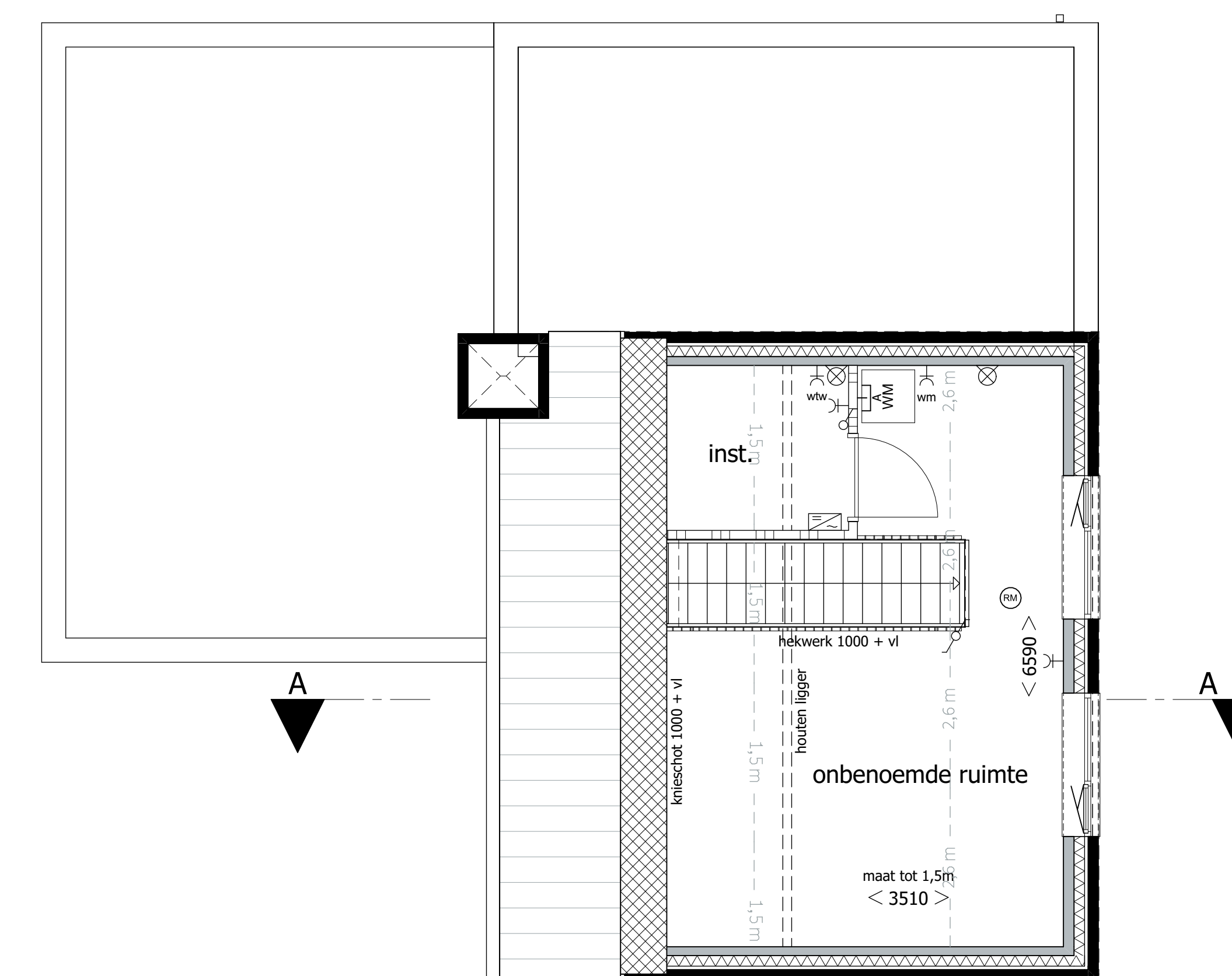
Verdieping 2 type C Bouwnummer 16 & 75
