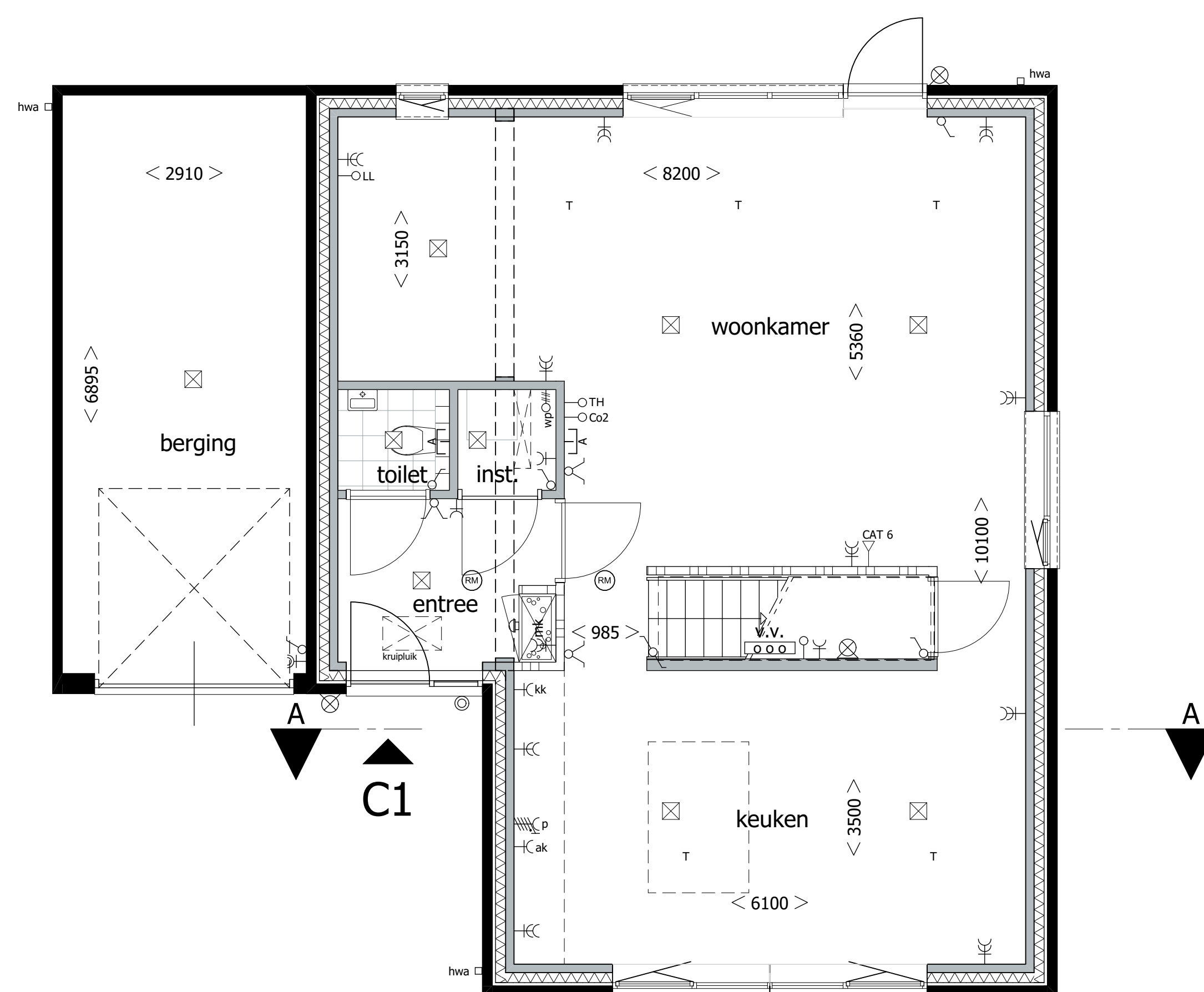
Begane grond type C Bouwnummer 16 & 75
