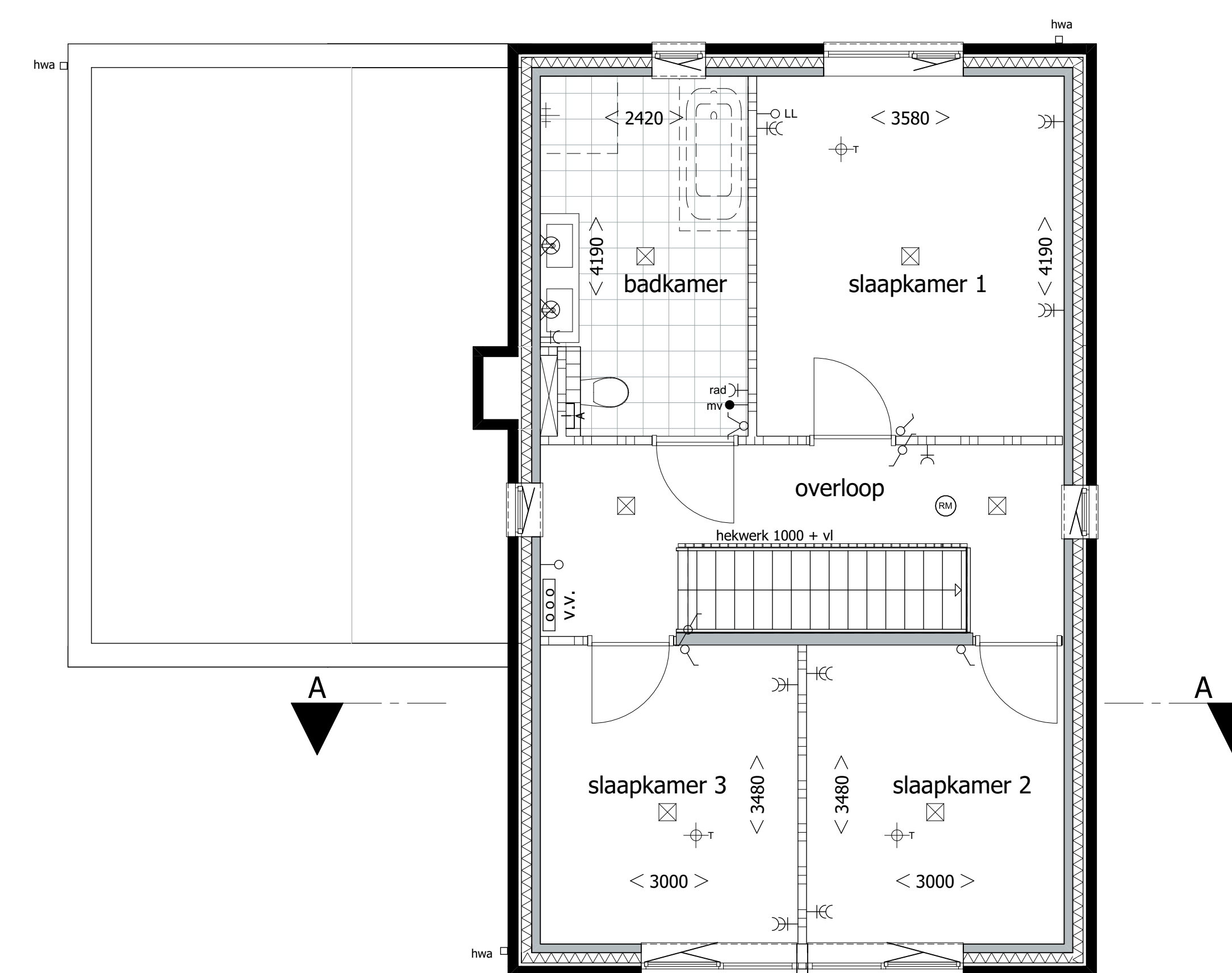
Verdieping 1 type C Bouwnummer 16 & 75
